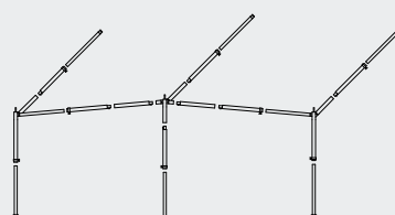
Frame Locarno Plus
